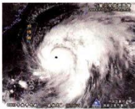
图 6.54 (b) 2008 年 9 月 11 日 1 时 25 分 卫星云图 (图片来源: 国家卫星气象中心)
