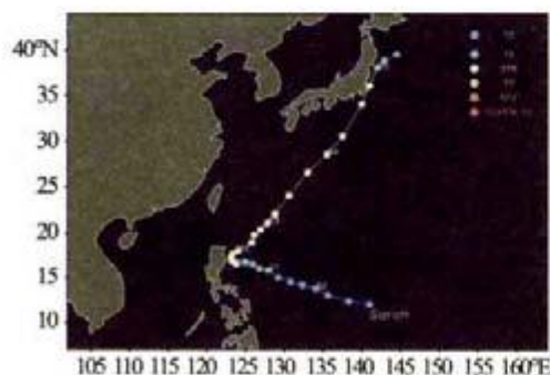
图 6.26 (a) 强热带风暴 Sarah (8611) 路径图
