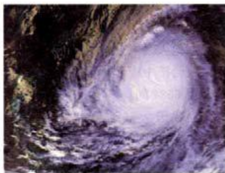
图 6.28 (b) 1987 年 10 月 21 日 05 时 15 分卫星云图
