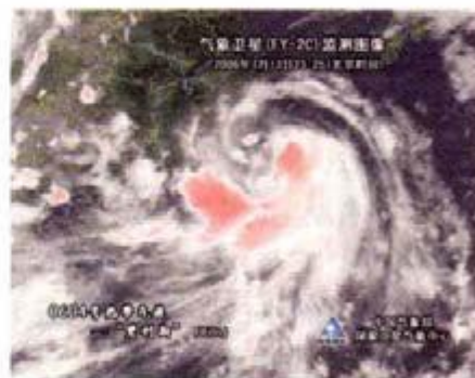
图 6.49 (b) 2006 年 7 月 13 日 23 时 25 分 FY-2C 云图 (图片来源：国家卫星气象中心)
