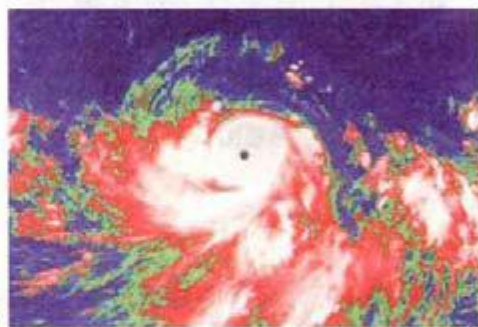
图 6.25 (b) 1986年7月7日11时 GMS-3 卫星云图
