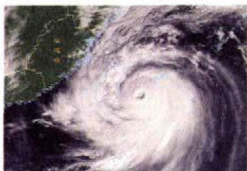
图 6.55 (c) 2008 年 9 月 28 日 10 时 25 分 FY-3A 云图 (图片来源: 国家卫星气象中心)
