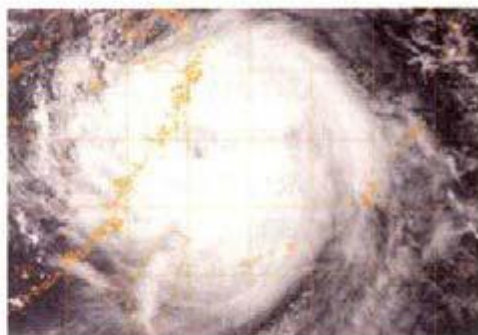
图 6.44 (b) 2004年8月12日14时 可见光云图 (图片来源: http://www.nrlmry.navy.mil )
