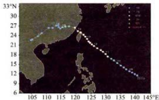
图 6.49 (a) 强热带风暴“碧利斯”(0604) 路径图
