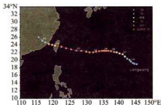
图 6.48 (a) 超强台风“龙王”(0519) 路径图
