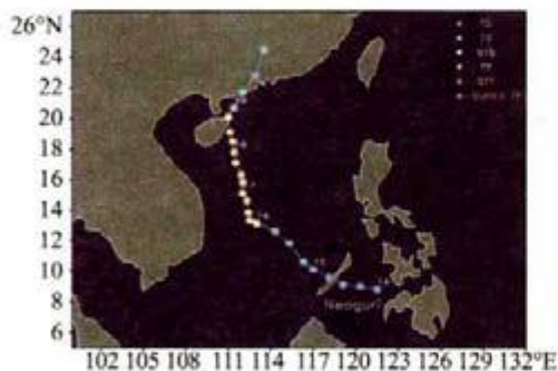
图 6.53 (a) 台风“浣熊”(0801) 路径图
