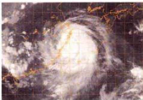
图 6.44 (c) “云娜”即将登陆时的红外云图 (图片来源: http://www.nrlmry.navy.mil )
