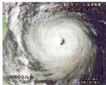
图 6.48 (b) 2005 年 10 月 1 日 06 时 36 分 FY-1D 云图
