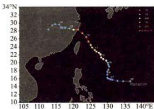
图 6.44 (a) 强台风“云娜”(0414) 路径图
