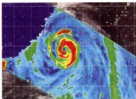
图 6.48 (e) “龙王”登陆台湾前的 TRMM 卫星云图 (图片来源: http://www.nrlmry.navy.mil )
