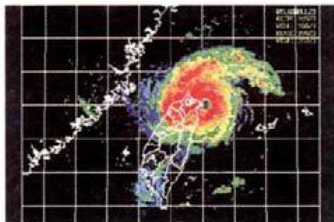
图 6.42 (c) “百合”登陆台湾前的雷达图像
