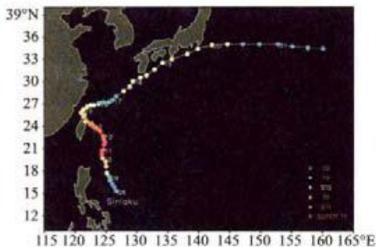
图 6.54 (a) 超强台风“森拉克”(0813) 路径图
