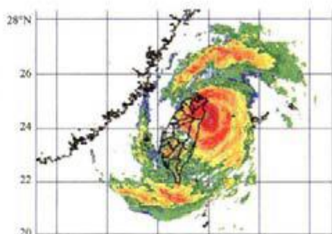
图 6.55 (d) “蔷薇”即将登陆台湾的 雷达图像 (图片来源: http://www.cwda.gov.tw/ )
