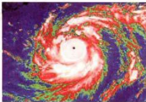
图 6.30 (b) 1989 年 7 月 15 日 11 时 GMS-3 卫星云图 (图片来源: http://agorn.ex.nui.ac.jp/ )
